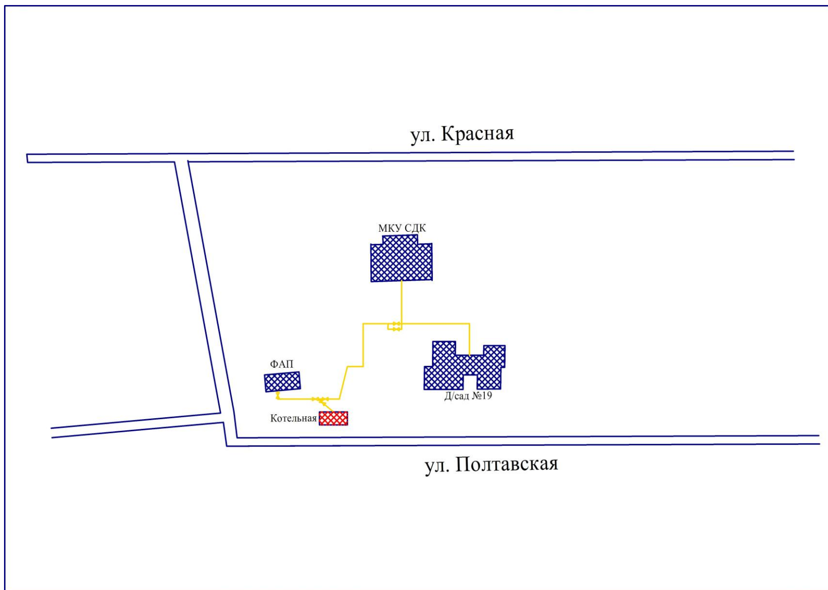
Рис 2. Схема теплоснабжения котельной МКУ СДК х. Куликовского
